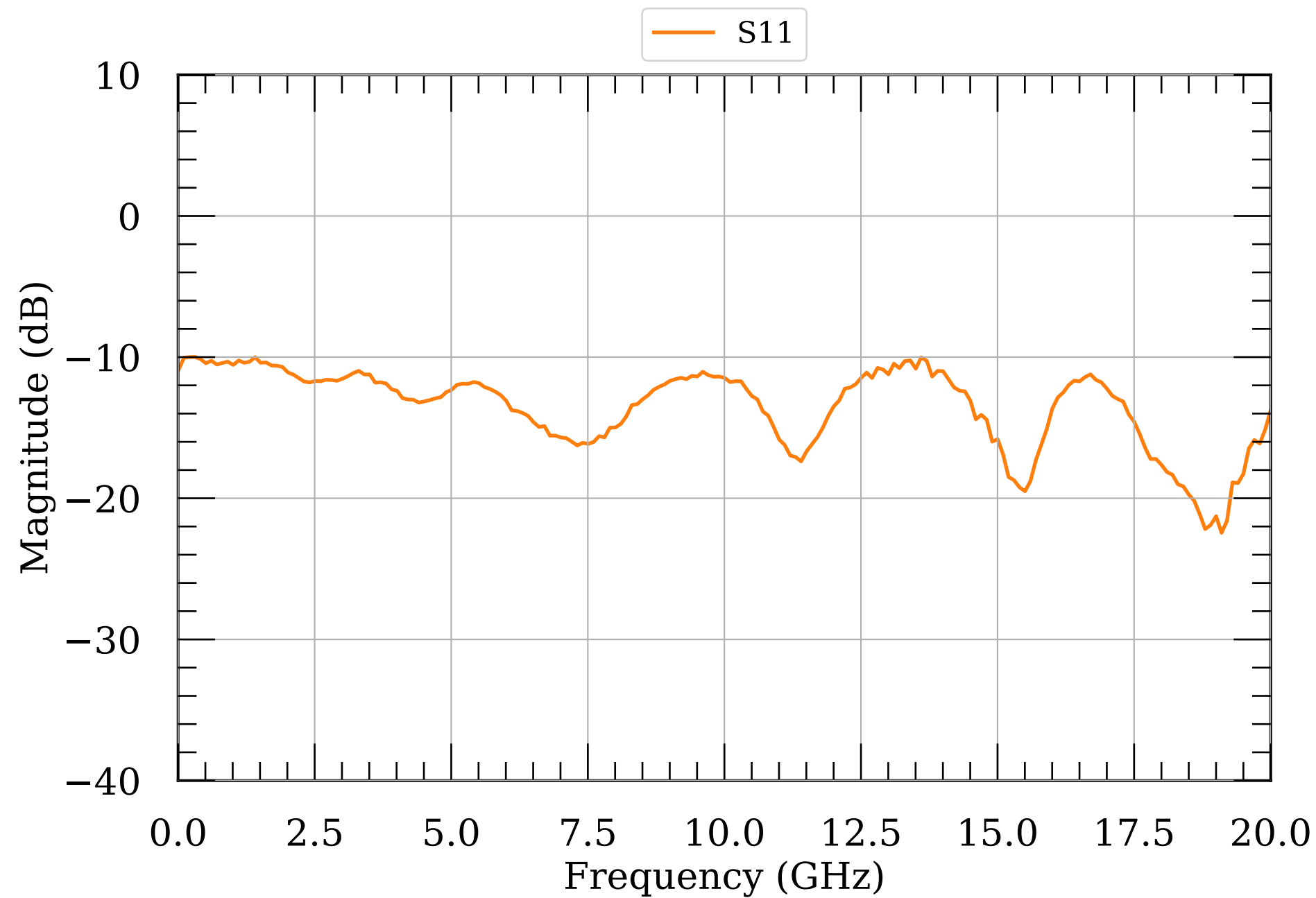
LNA S-params module047
